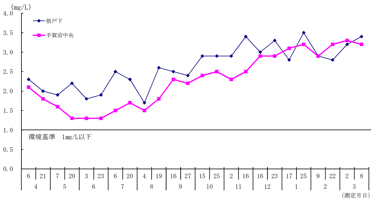
図1-9 手賀沼の全窒素の月別変化（令和3年度）
