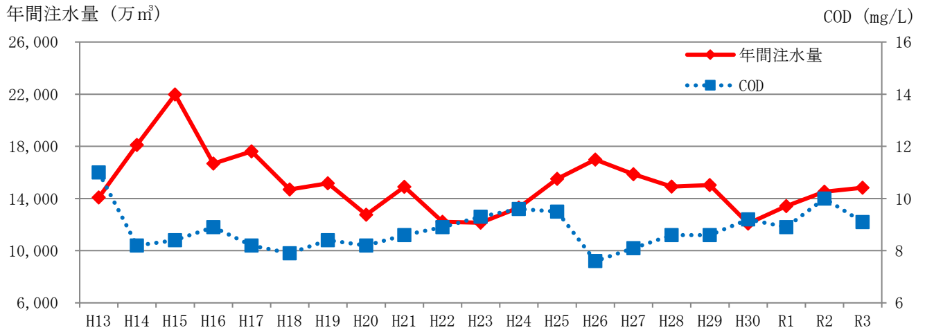
図1-14 北千葉導水年間注水量及びCOD
