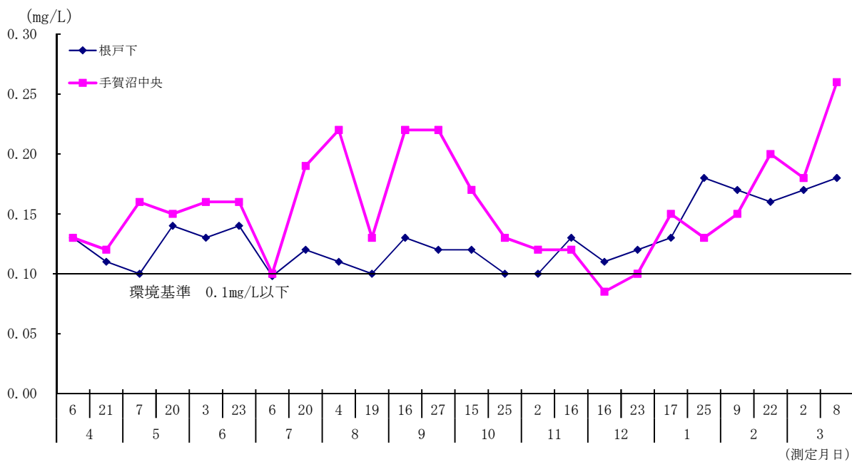
図1-10 手賀沼の全リンの月別変化（令和3年度）
