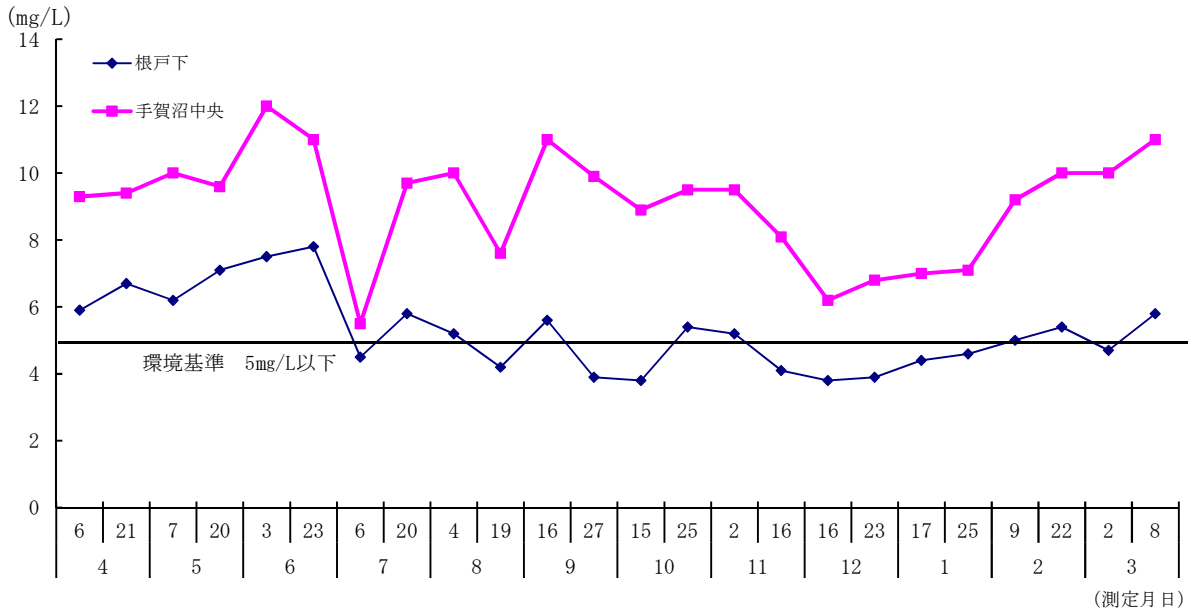
図1-8 手賀沼のCODの月別変化（令和3年度）
