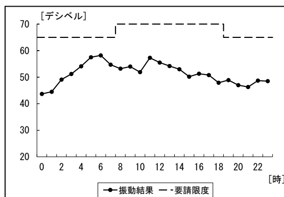
図 5-2-2 振動レベル経時変化
