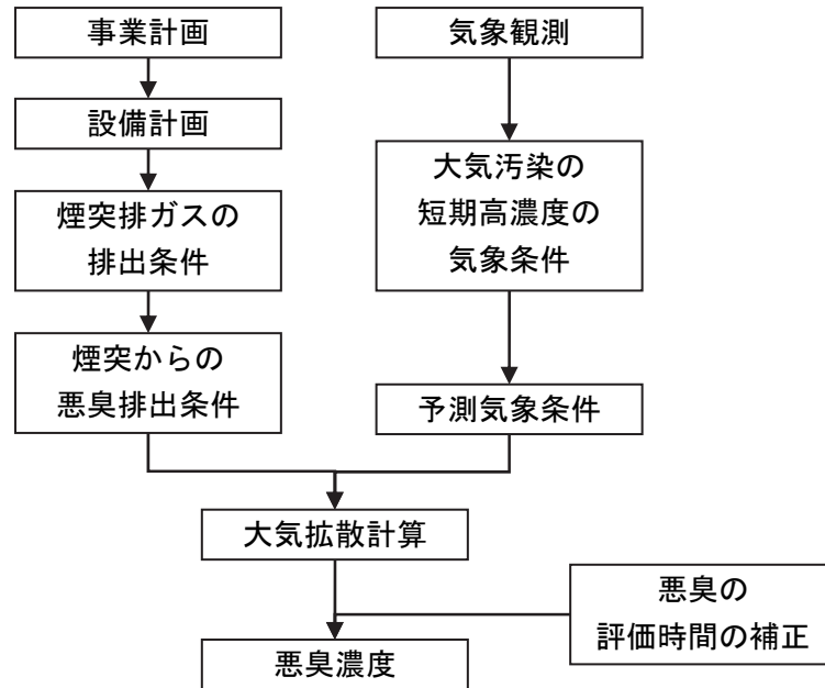
図 7-2-91 新廃棄物処理施設の稼働（煙突排出ガス）による影響の予測手順
