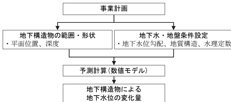
図 7-2-46 新廃棄物処理施設及びリサイクルセンターの存在による地下水位の変化の予測手順
