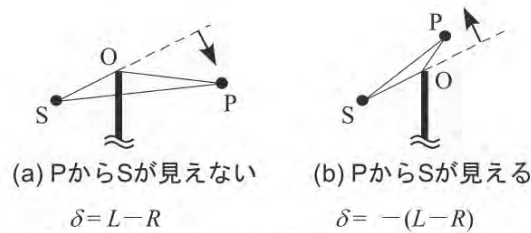
図-3.1 直達経路 R = SP , 回折経路 L = SO + OP , 回折経路差 \delta の定義
