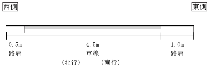
図 7-2-84(4) 道路横断面構成 (T4 (新木野団地))
