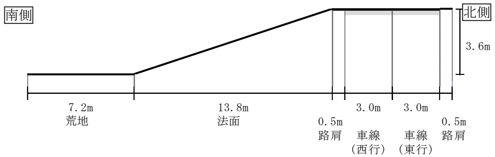
図 7-2-84(2) 道路横断面構成 (T2 (江蔵地))
