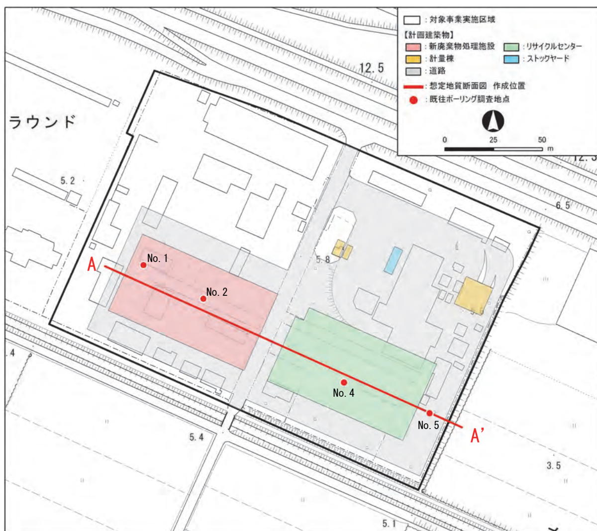
図 7-2-93 地質想定断面図の作成位置
