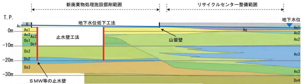
図 7-2-41 地下構造物の設置等に伴う掘削工事範囲 (新廃棄物処理施設)
