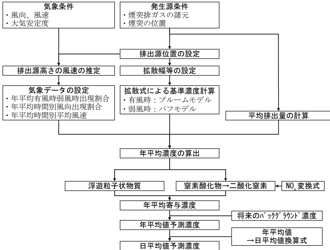
図 7-2-21 新廃棄物処理施設の稼働による大気質（長期平均濃度）の予測手順
