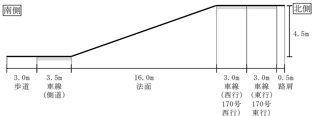
図 7-2-26(1) 道路横断面構成 (T1 (つつじ荘前))
