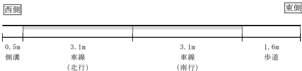
図 7-2-26(3) 道路横断面構成（T3（吾妻処理場））
