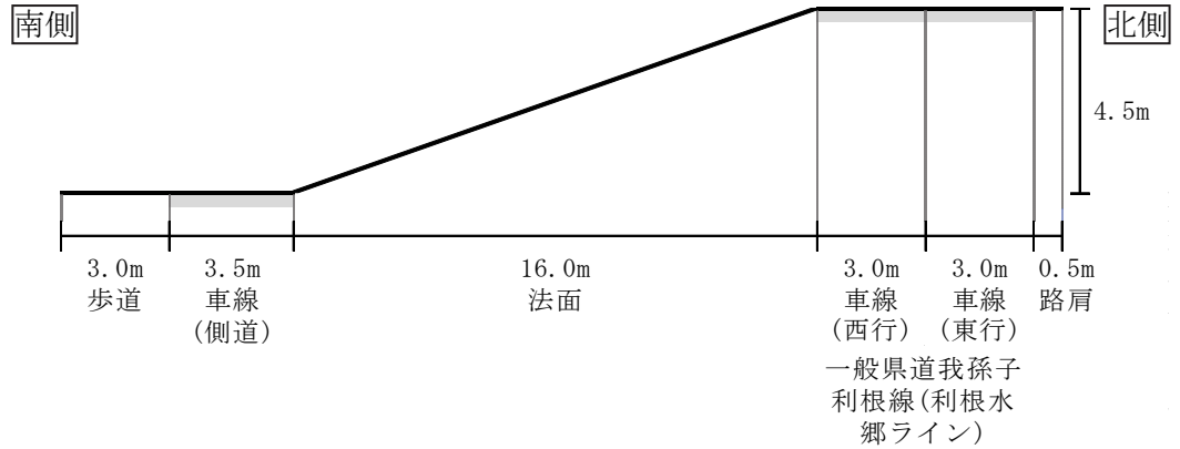
図 7-2-67(1) 道路横断面構成 (T1 (つっじ荘前))
