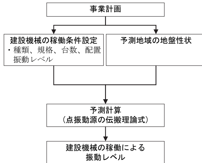
図 7-2-72 建設機械の稼働による振動の予測手順
