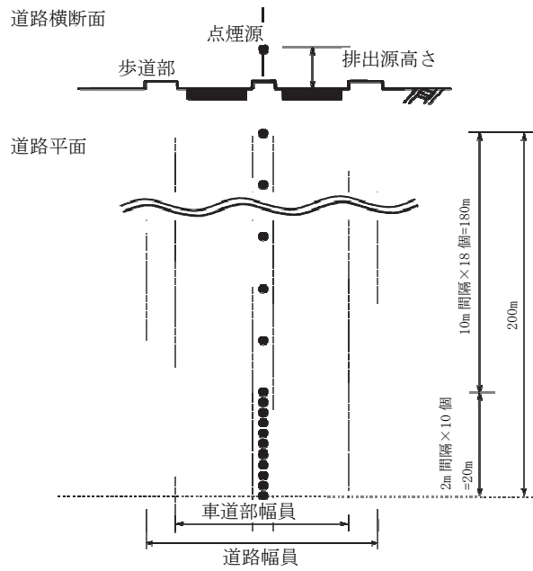
図 7-2-11 煙源の配置
