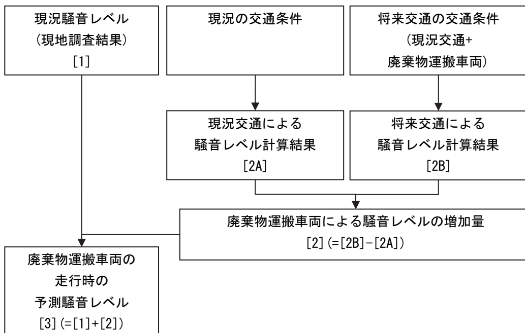
図 7-2-69 廃棄物運搬車両の走行による道路交通騒音の予測手順
