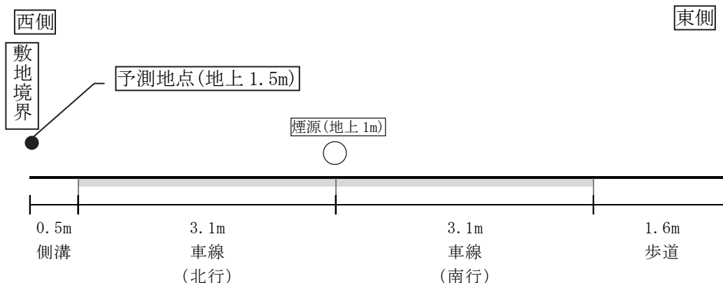
図 7-2-30(3) 予測地点道路断面図 (T3 (吾妻処理場))
