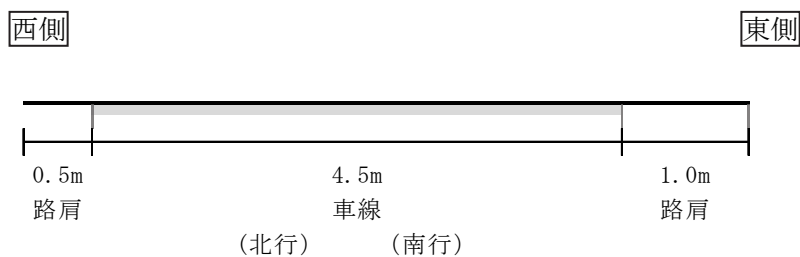
図 7-2-26(4) 道路横断面構成（T4（新木野団地））
