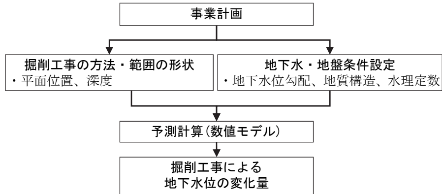
図 7-2-40 工事の実施による地下水位の変化の予測手順
