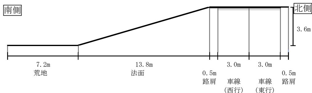
図 7-2-26(2) 道路横断面構成 (T2 (江蔵地))
