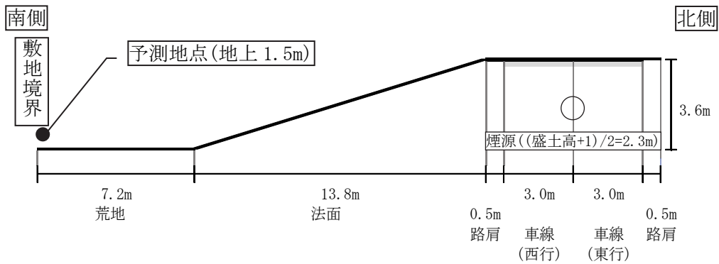
図 7-2-12(2) 予測地点道路断面図 (T2 (江蔵地))
