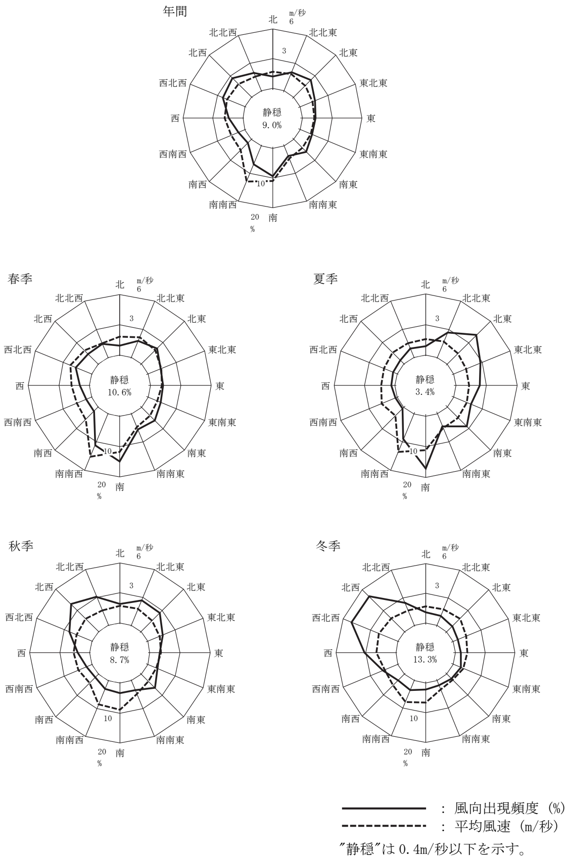
図 7-2-90 風配図
