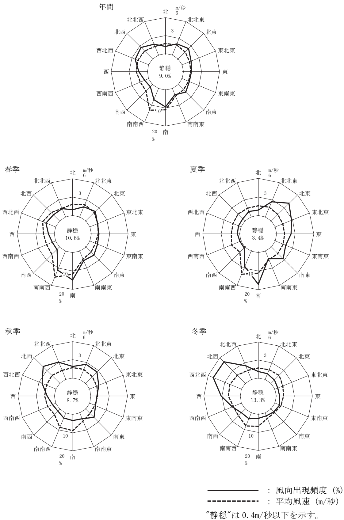
図 7-2-15 風配図
