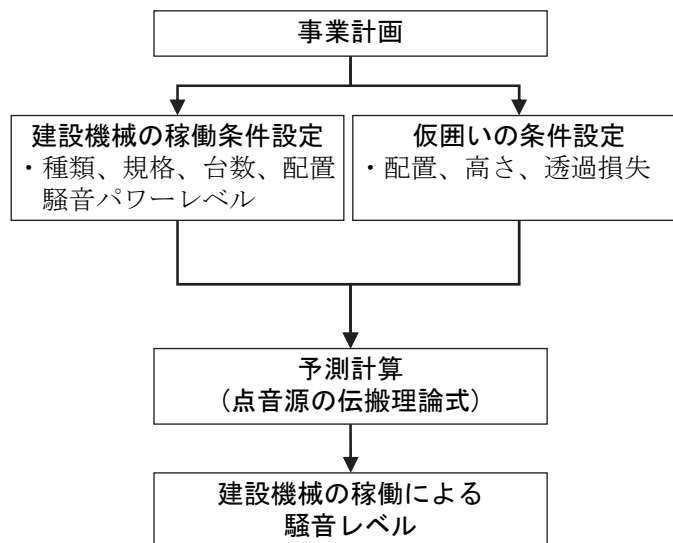
図 7-2-52 建設機械の稼働による騒音レベルの予測手順
