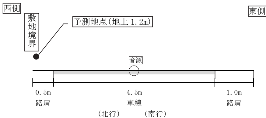
図 7-2-70(3) 予測地点道路断面図 (T3 (吾妻処理場))
