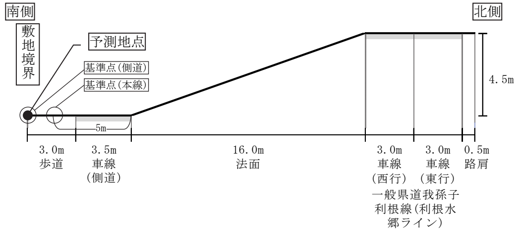
図 7-2-79(1) 予測地点道路断面図 (T1 (つつじ荘前))
