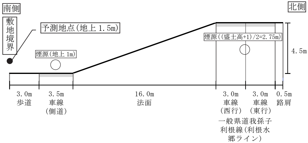
図 7-2-30(1) 予測地点道路断面図 (T1 (つつじ荘前))
