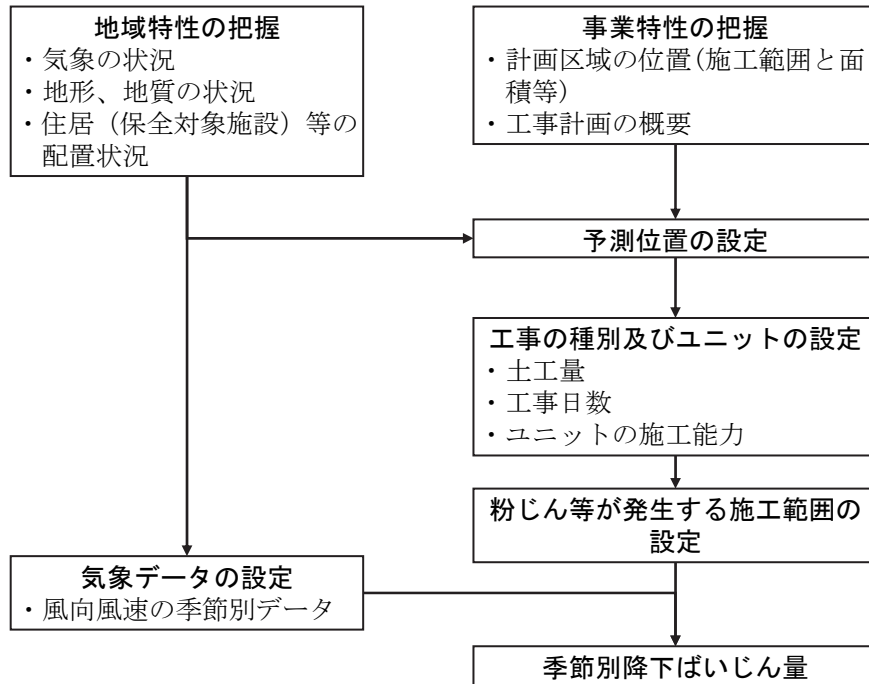
図 7-2-4 予測手順(降下ばいじん量)
