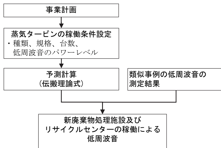
図 7-2-64 新廃棄物処理施設及びリサイクルセンターの稼働による低周波音の予測手順
