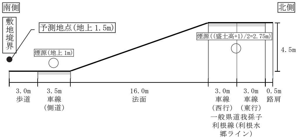
図 7-2-12(1) 予測地点道路断面図 (T1 (つつじ荘前))
