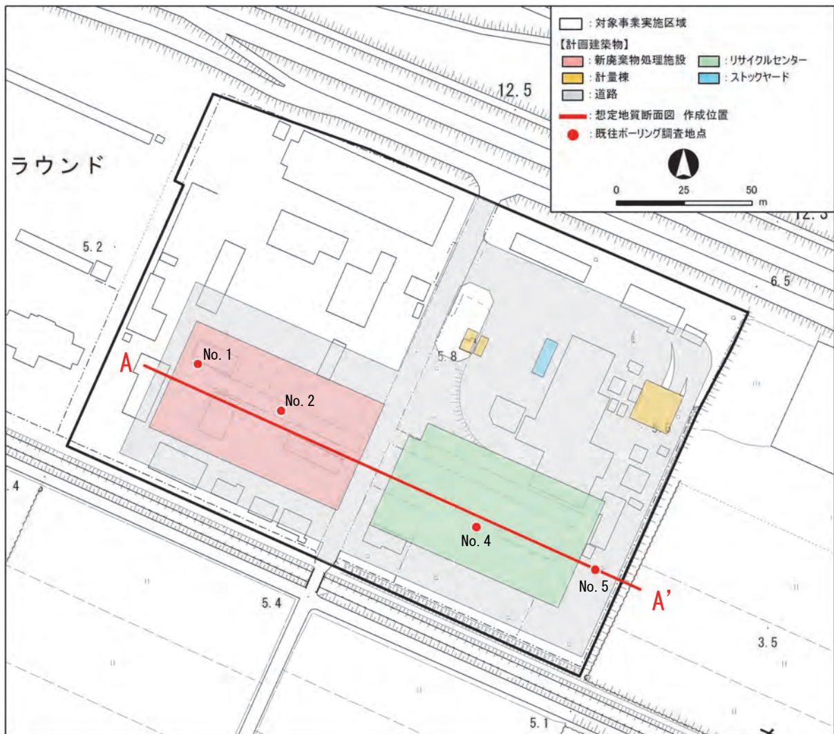
図 7-2-99 地質想定断面図の作成位置
