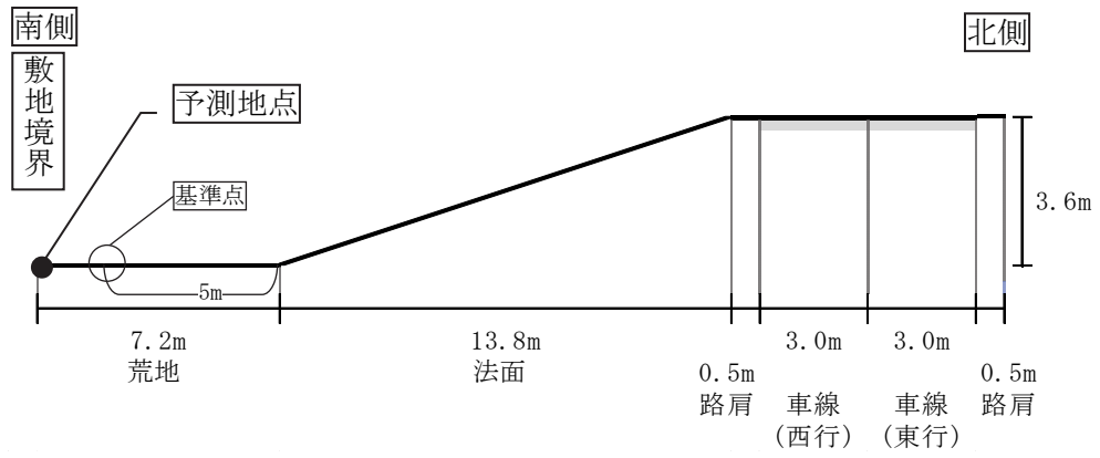
图 7-2-87(2) 予測地点道路断面图 (T2 (江蔵地))
