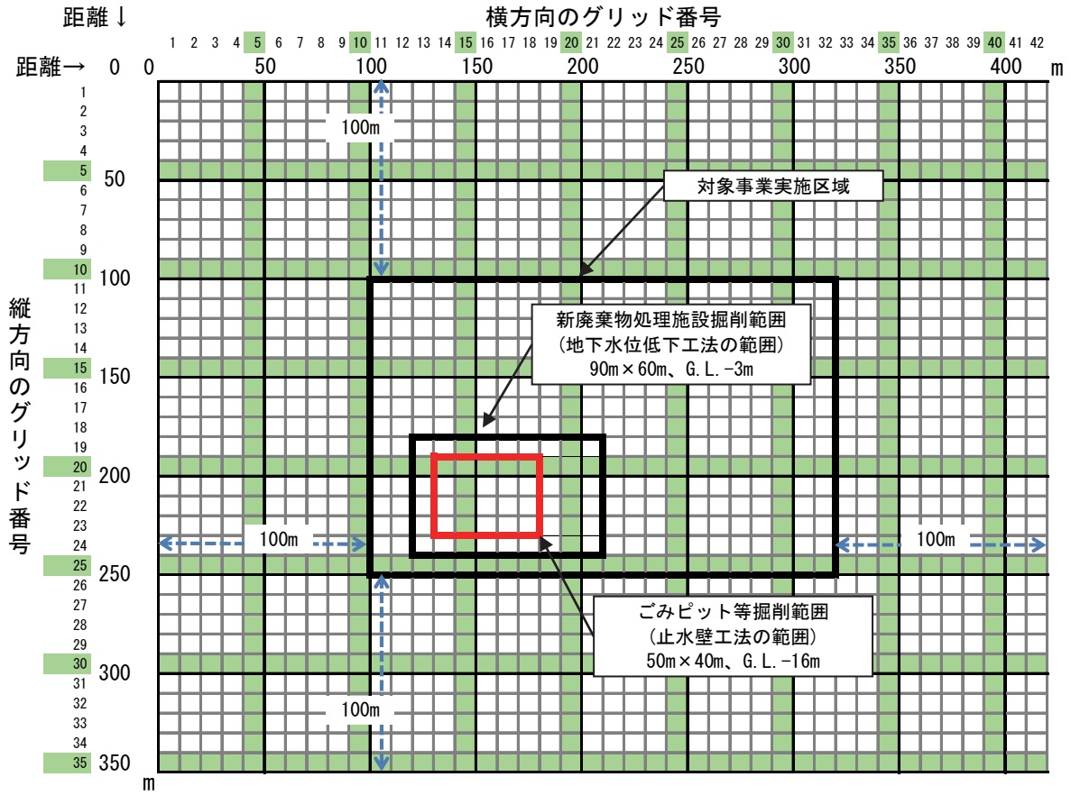
図 7-2-42 平面配置 (工事の実施)
