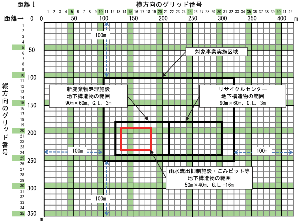
図 7-2-48 平面配置（新廃棄物処理施設及びリサイクルセンターの存在）
