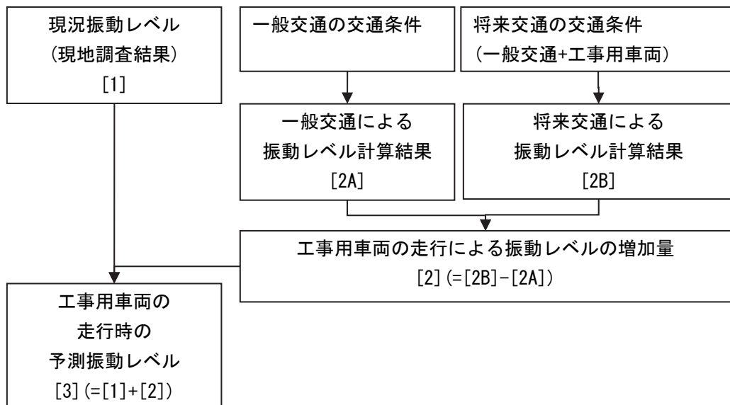
図 7-2-78 工事用車両の走行による振動の予測手順
