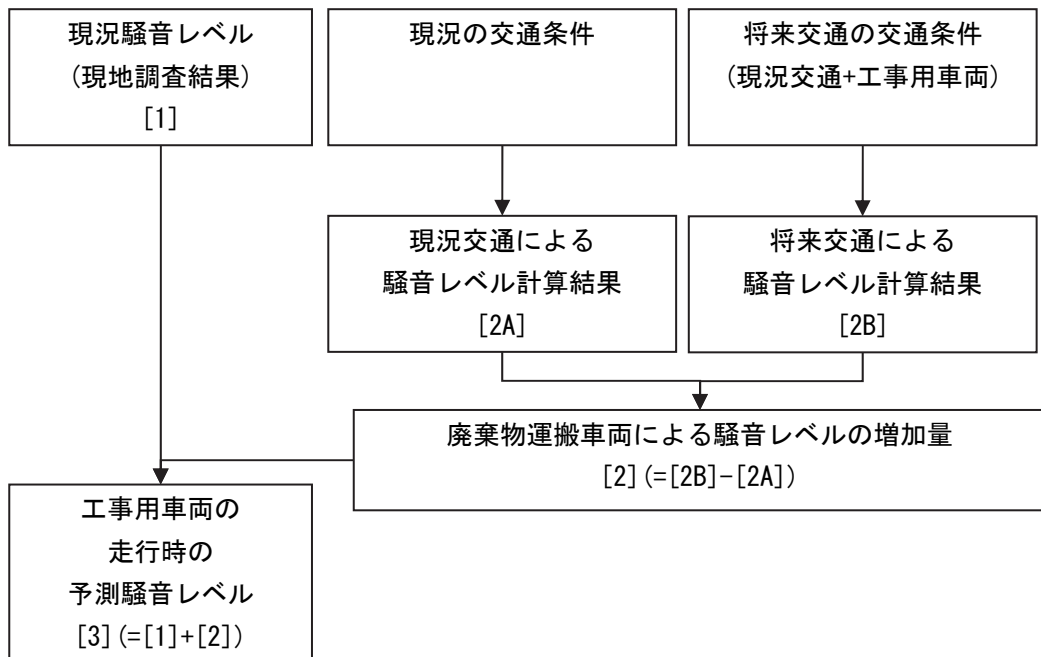
図 7-2-58 工事用車両の走行による道路交通騒音の予測手順
