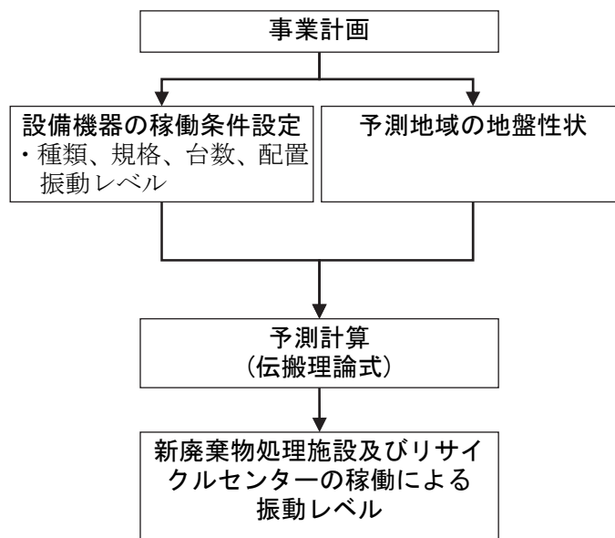
図 7-2-81 新廃棄物処理施設の稼働による振動の予測手順
