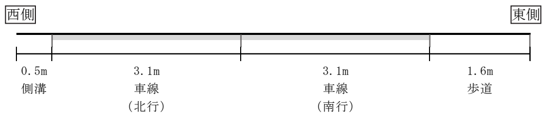
図 7-2-67(3) 道路横断面構成 (T3 (吾妻処理場))
