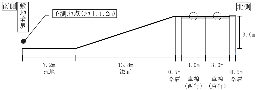
図 7-2-59(2) 予測地点道路断面図 (T2 (江蔵地))
