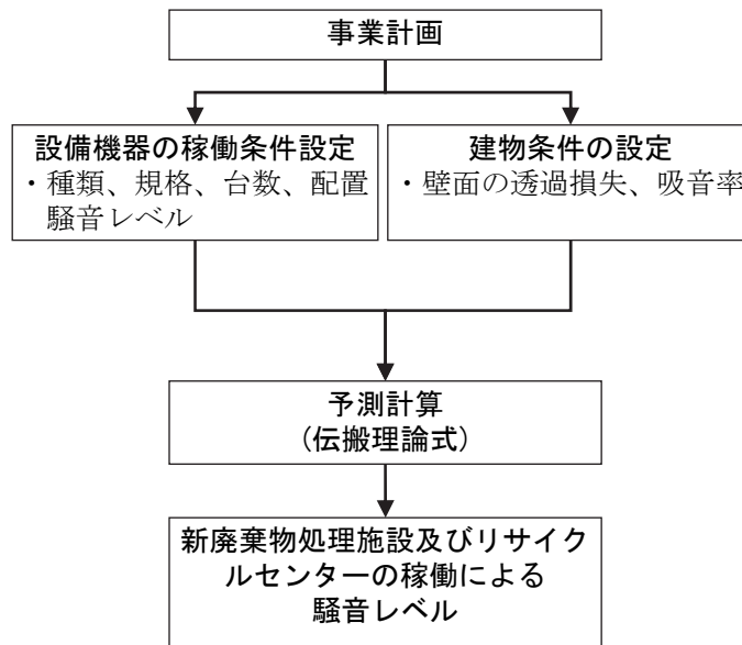
図 7-2-61 新廃棄物処理施設稼働による騒音の予測手順
