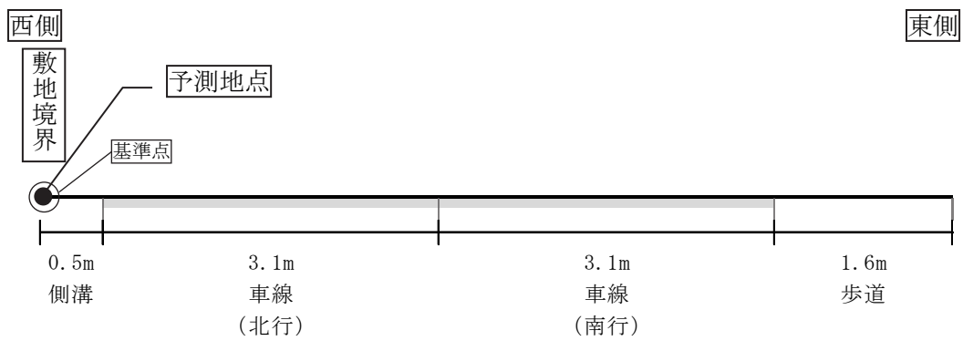
图 7-2-87(3) 予測地点道路断面图 (T3 (吾妻処理場))
