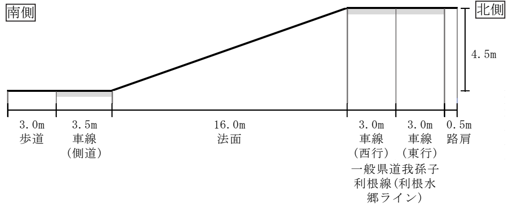
図 7-2-84(1) 道路横断面構成 (T1 (つつじ荘前))
