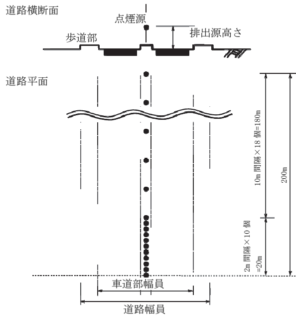
図 7-2-29 煙源の配置
