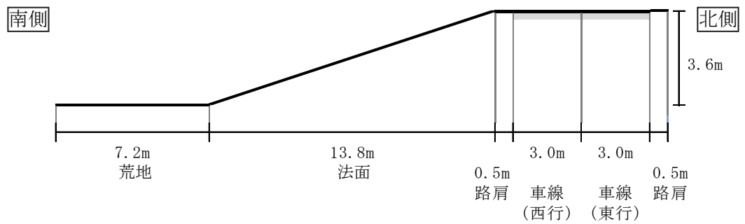
図 7-2-67(2) 道路横断面構成 (T2 (江蔵地))
