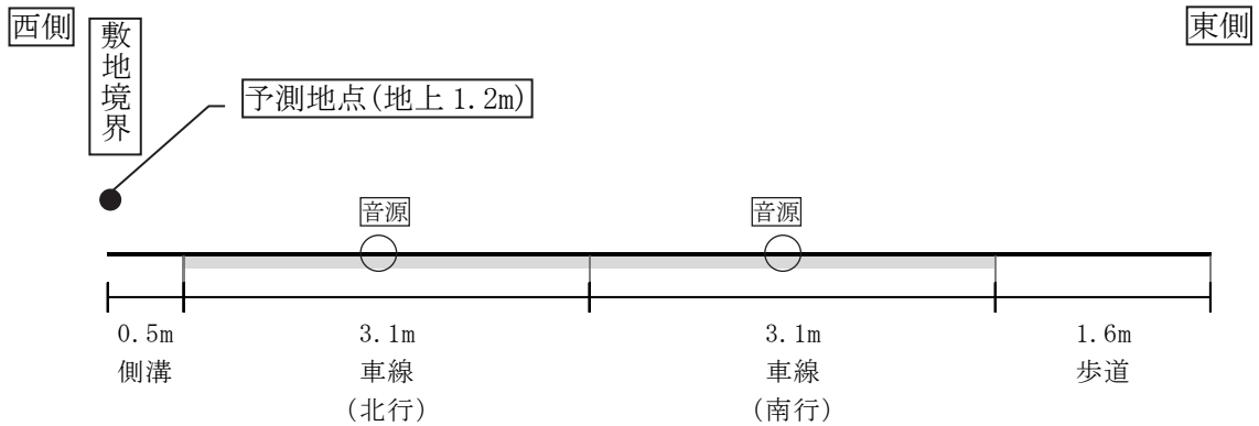
図 7-2-70(3) 予測地点道路断面図 (T3 (吾妻処理場))
