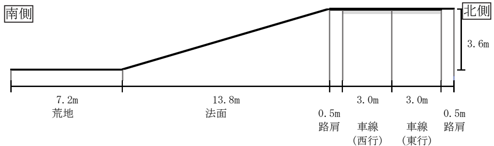
図 7-2-8(2) 道路横断面構成 (T2 (江蔵地))
