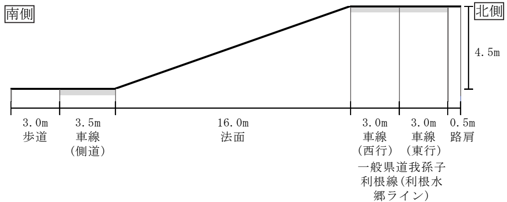
図 7-2-8(1) 道路横断面構成 (T1 (つつじ荘前))
