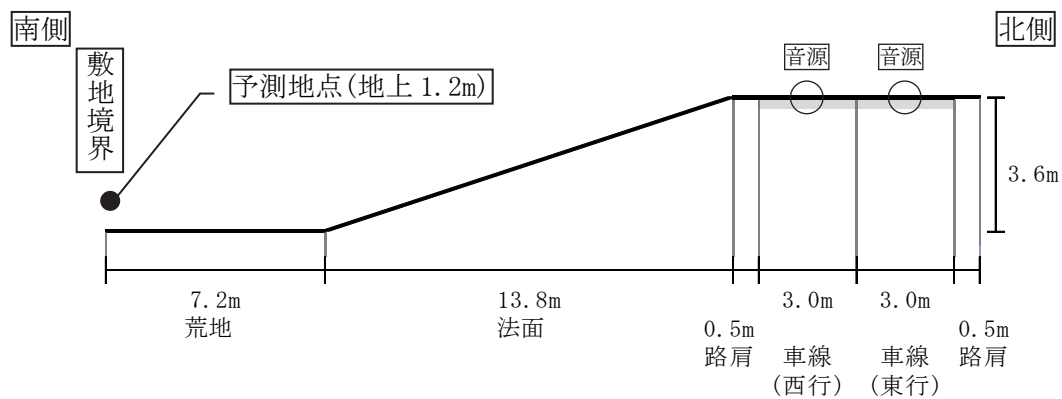
図 7-2-70(1) 予測地点道路断面図 (T1 (つつじ荘前))
