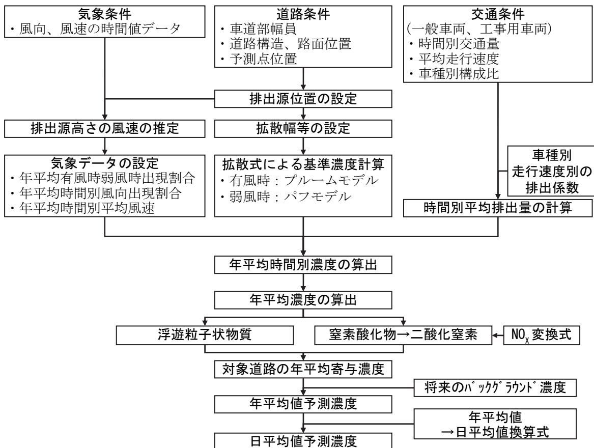
図 7-2-10 工事用車両の走行による沿道大気質の予測手順
