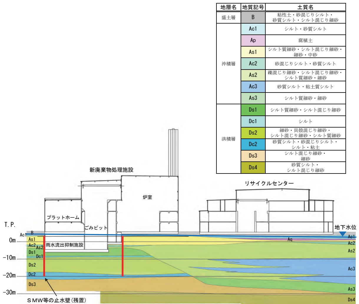
図 7-2-47 地下構造物範囲 (新廃棄物処理施設及びリサイクルセンター)
