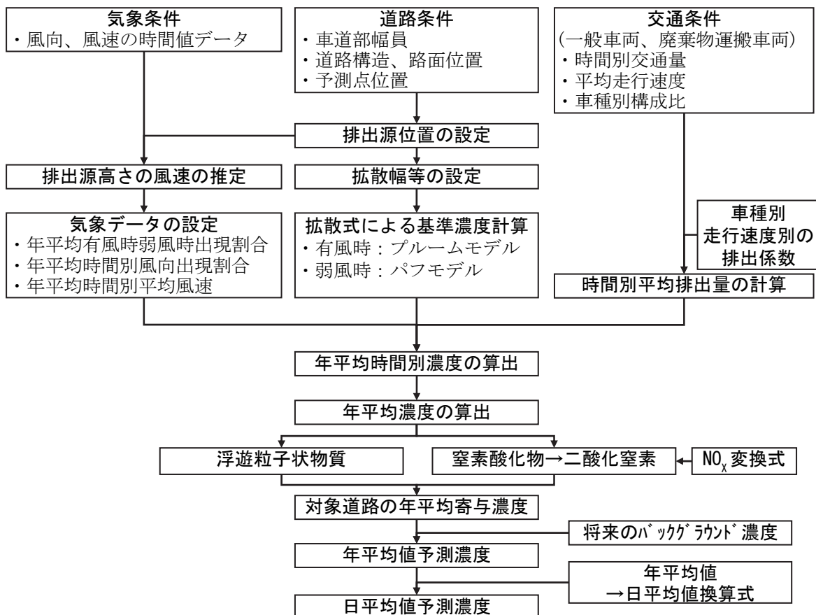
図 7-2-28 廃棄物運搬車両の走行による沿道大気質の予測手順
