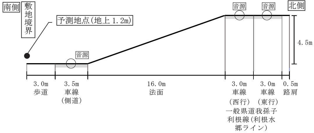
図 7-2-59(1) 予測地点道路断面図 (T1 (つつじ荘前))
