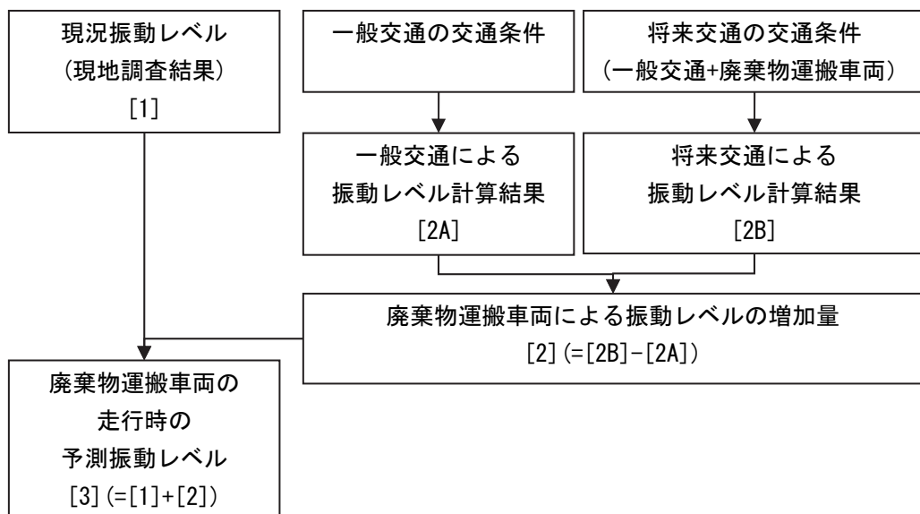
図 7-2-86 廃棄物運搬車両の走行による道路交通振動の予測手順
