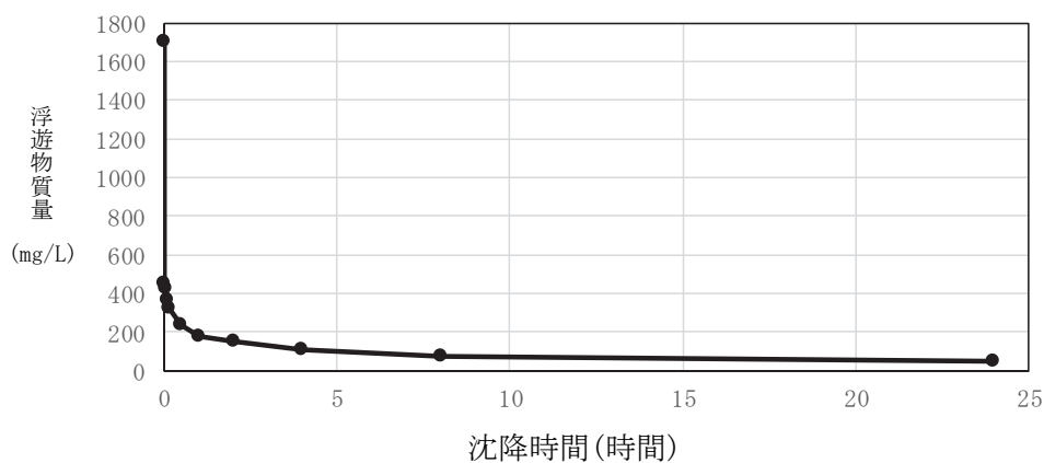
図 7-2-34 土壌沈降試験結果
