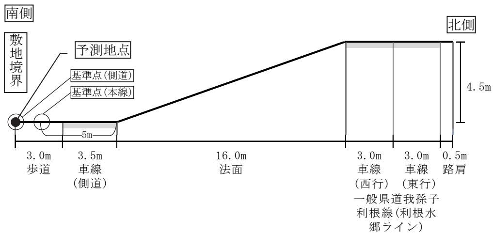
図 7-2-87(1) 予測地点道路断面図 (T1 (つつじ荘前))
