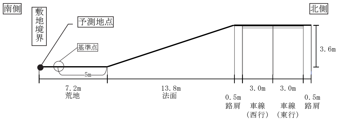
図 7-2-79(2) 予測地点道路断面図 (T2 (江蔵地))
