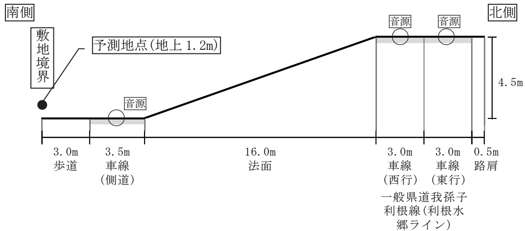
図 7-2-70(1) 予測地点道路断面図 (T1 (つつじ荘前))
