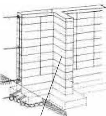
控壁：高さが1.2mを超えるブロック塀は、3.4m以内の間隔で設置が必要
