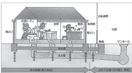
下水を運ぶ方式には、汚水と雨水を1本の管で運ぶ合流式と、別々の管で運ぶ分流式があり、我孫子市では分流式を採用しています。
