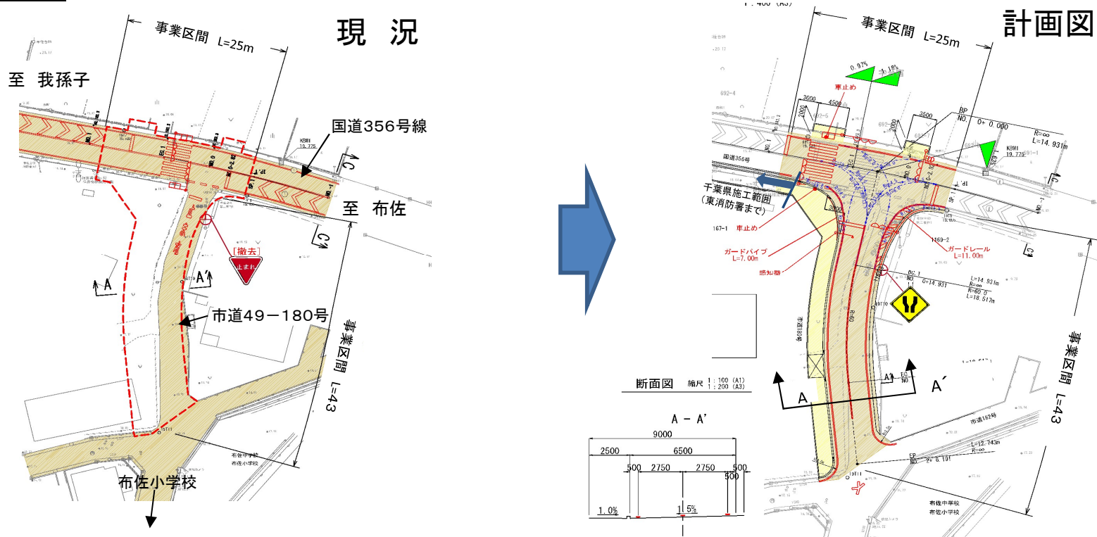
○市事業範囲計画図
